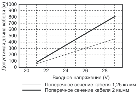
Напряжение питания и длина кабеля для источника питания кода 2
