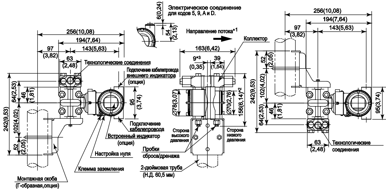
Рабочий штуцер вверх (Код монтажа 6)
