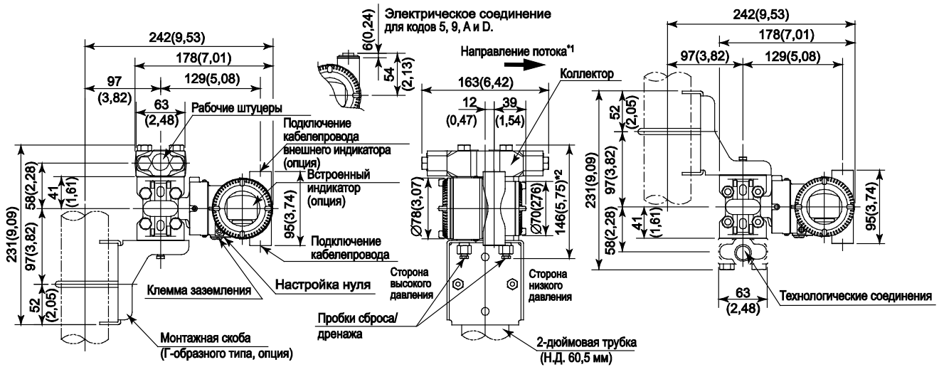
Рабочий штуцер вниз (Код монтажа 7)
