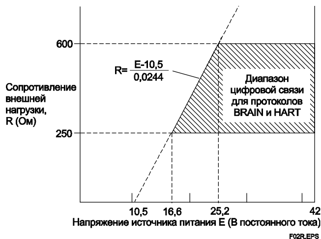
Рисунок 2. Взаимосвязь между напряжением источника питания и сопротивлением внешней нагрузки (Выходной сигнал с кодами D и J)
