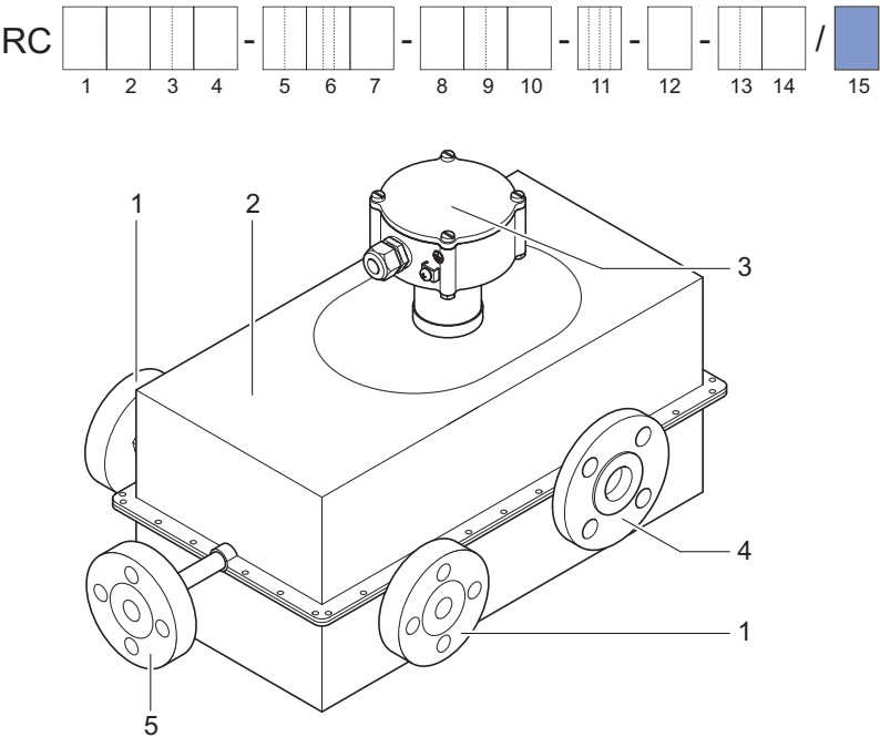
Рис. 21. Конфигурация Rotamass с изоляцией и обогревом линий
