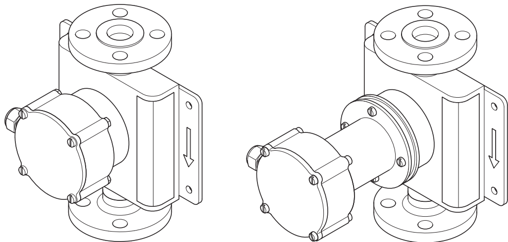
Рис. 25. Датчик со стандартным и удлиненным соединением
