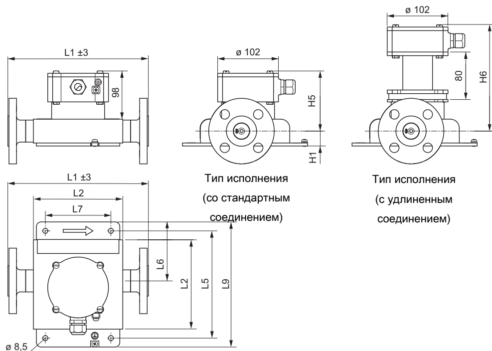
Рис. 26. Размеры в мм
