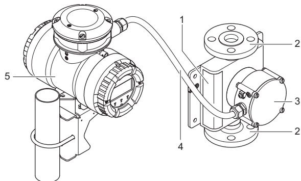
Рис. 5. Конфигурация разнесенного исполнения Rotamass
