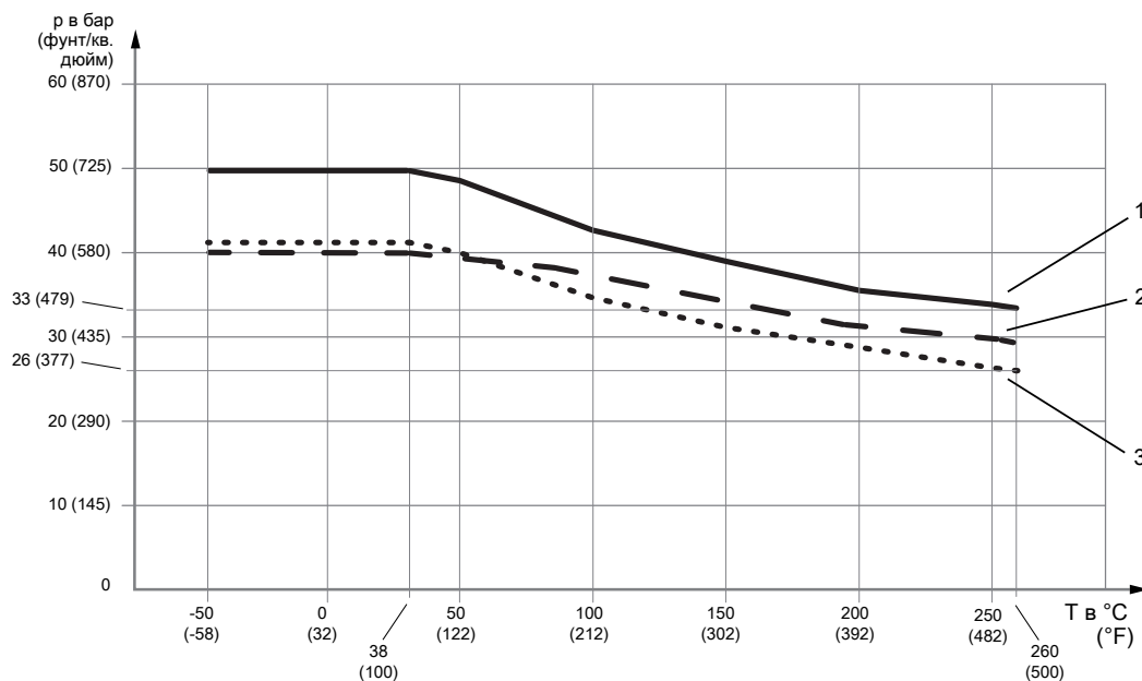
Рис. 13. Допустимое давление технологического процесса в зависимости от температуры в месте соединения с технологическим процессом
