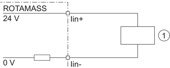
Рис. 46. Подсоединение внешнего устройства с пассивным токовым выходом
