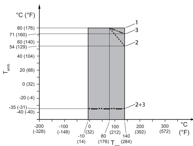
Рис. 25. Допустимая температура рабочей среды и окружающей среды, разнесенное исполнение, для типа присоединения к технологическому процессу HS4 и HS8
